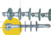
Aisladores de Vidrio y Sintetico.
